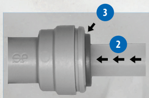
Wsuń powierzchnię czołową rurki LLDPE w gniazdo złącza wtykowego do samego końca (2). Pierścień zabezpieczający złączki wtykowej oprze się o korpus złącza wtykowego (3).
