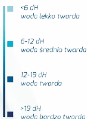
RYS. TWARDOŚĆ WODY W POLSCE
